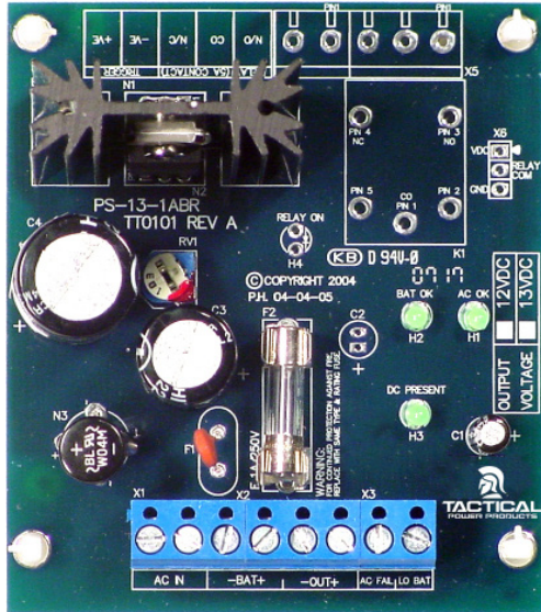
PS13-1A MODULE
