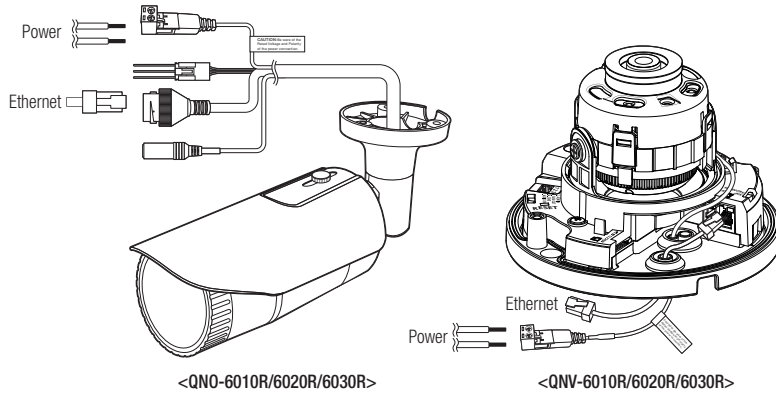
<QNO-6010R/6020R/6030R>
