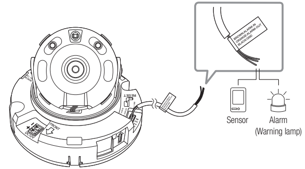
<QND-6010R/6020R/6030R>
