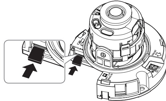
<QND-6010R/6020R/6030R>
