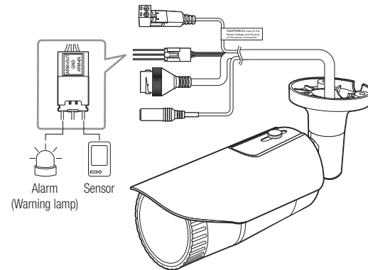
<QNO-6010R/6020R/6030R>
