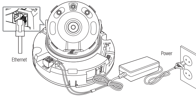
<QND-6010R/6020R/6030R>
